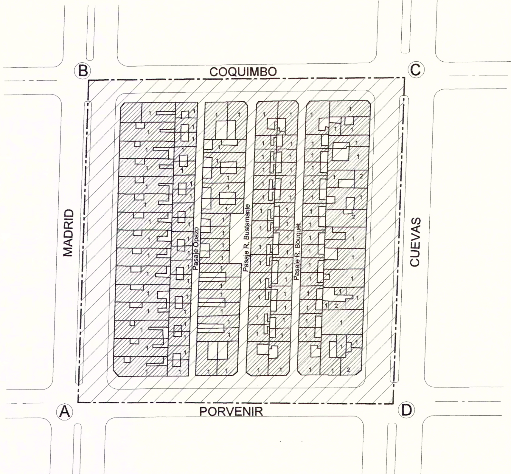
PLANO DE EMPLAZAMIENTO Esc. 1 : 1000
