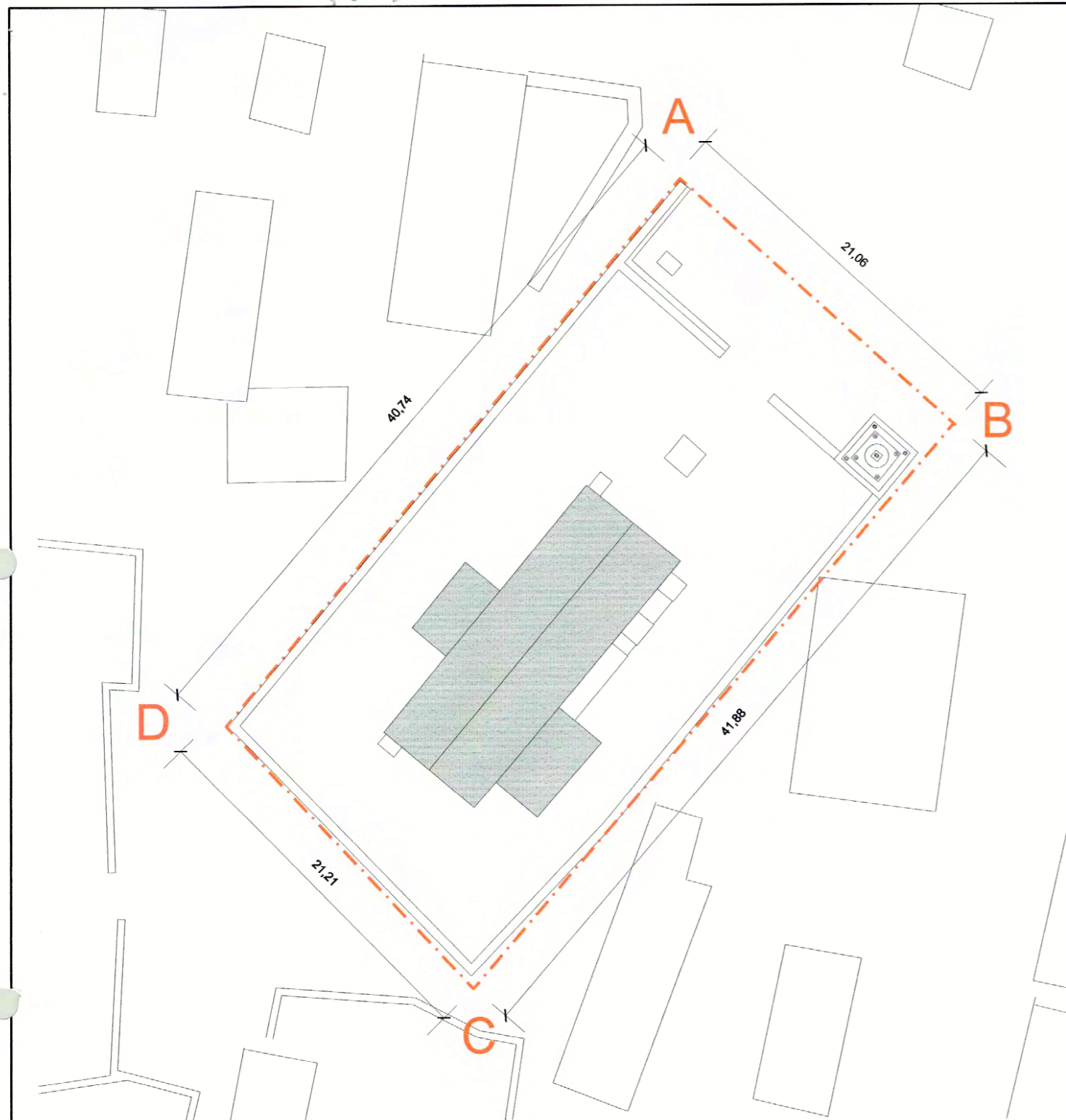
PLANO DE LIMITES escala 1:400
