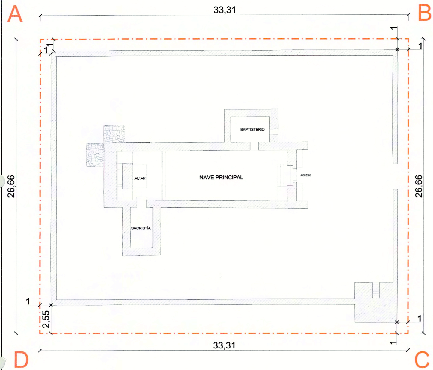
PLANO DE LIMITES escala 1:200
