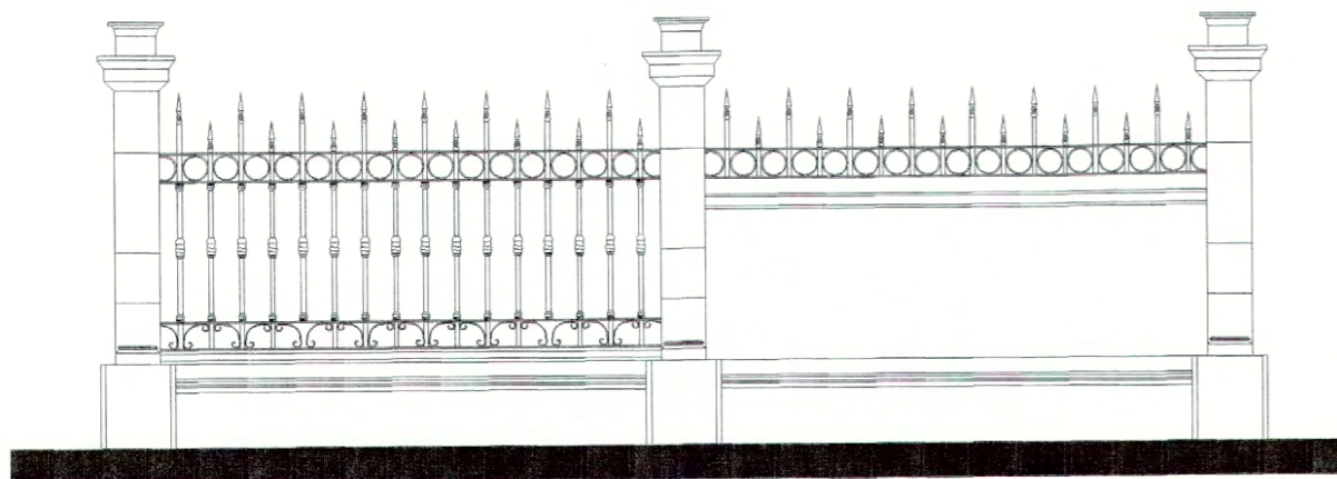
Detalle cierre exterior reja y muro lleno Av. Gran Avenida José Miguel Carrera ESC. 1 / 50
