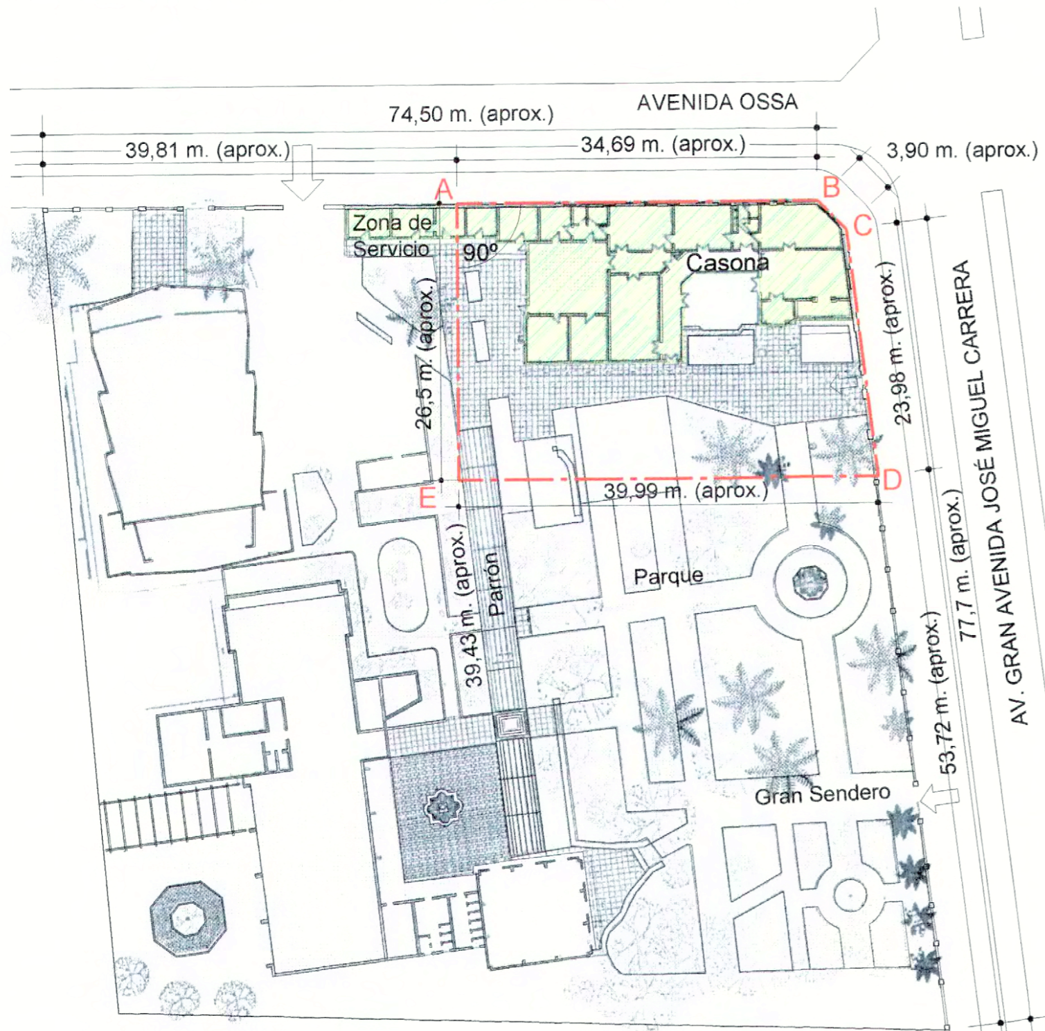
PLANTA GENERAL DE LÍMITES ESC. 1 / 500
