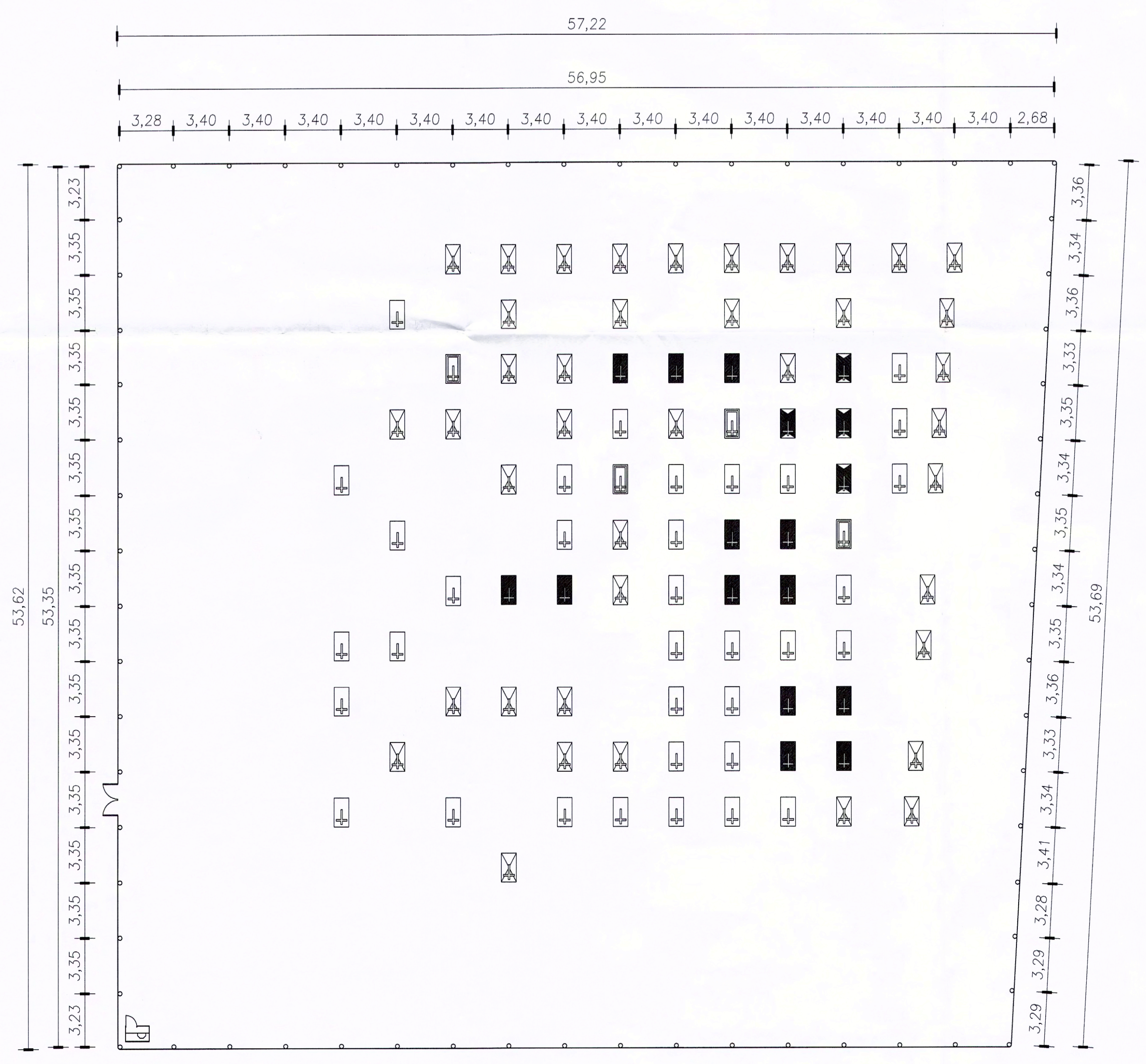
PLANTA DEL ELTUWE (CEMENTERIO) ESC. 1/200
