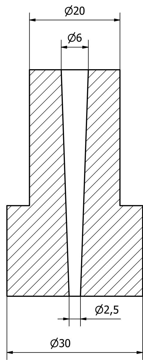
A-A ( 2 : 1 )
